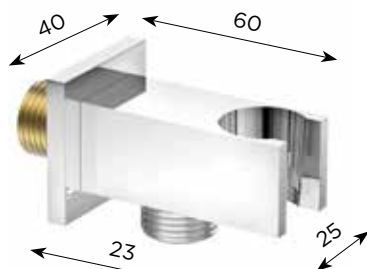
SALIDA FLEXO MURAL CON SOPORTE CUADRADO
